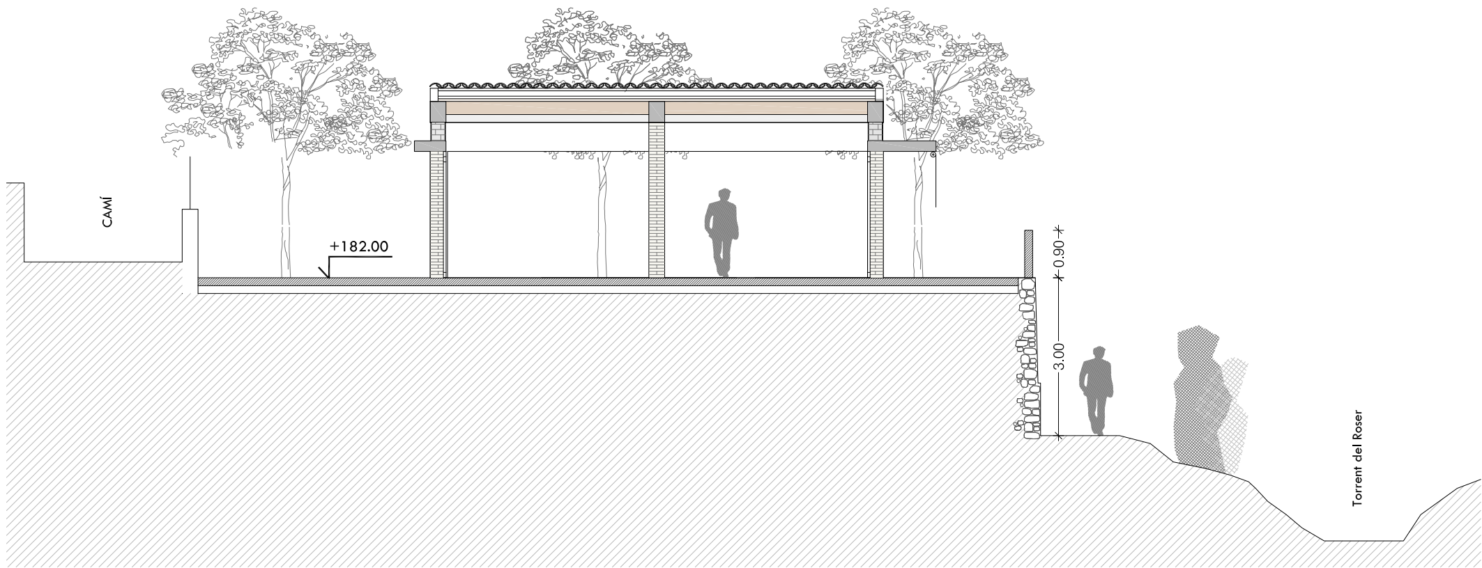
SECCIÓ 2
