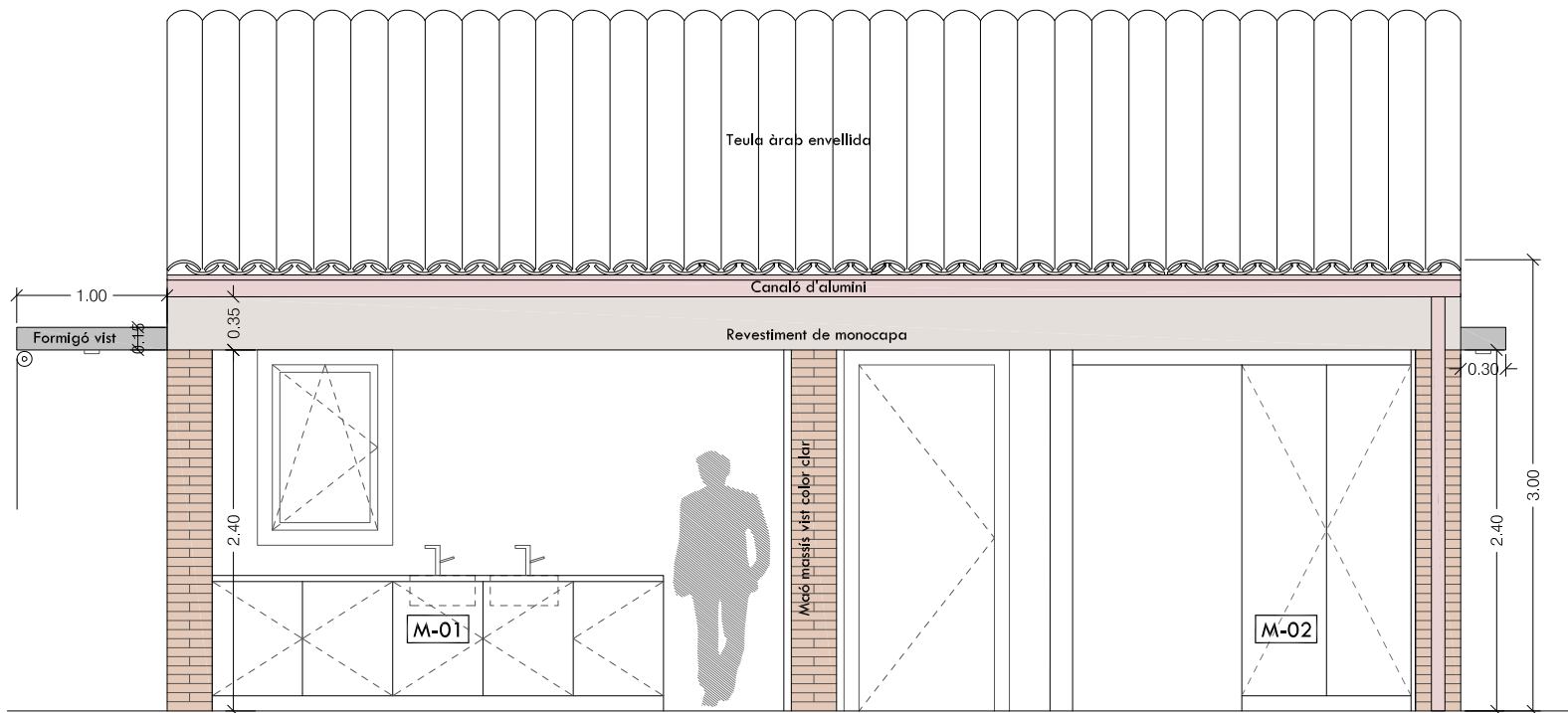
ALÇAT EST
