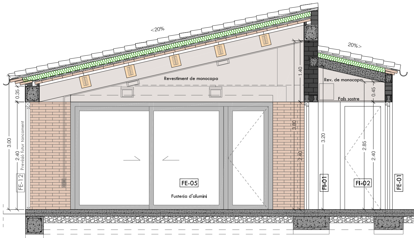
SECCIÓ TRANSVERSAL 1
