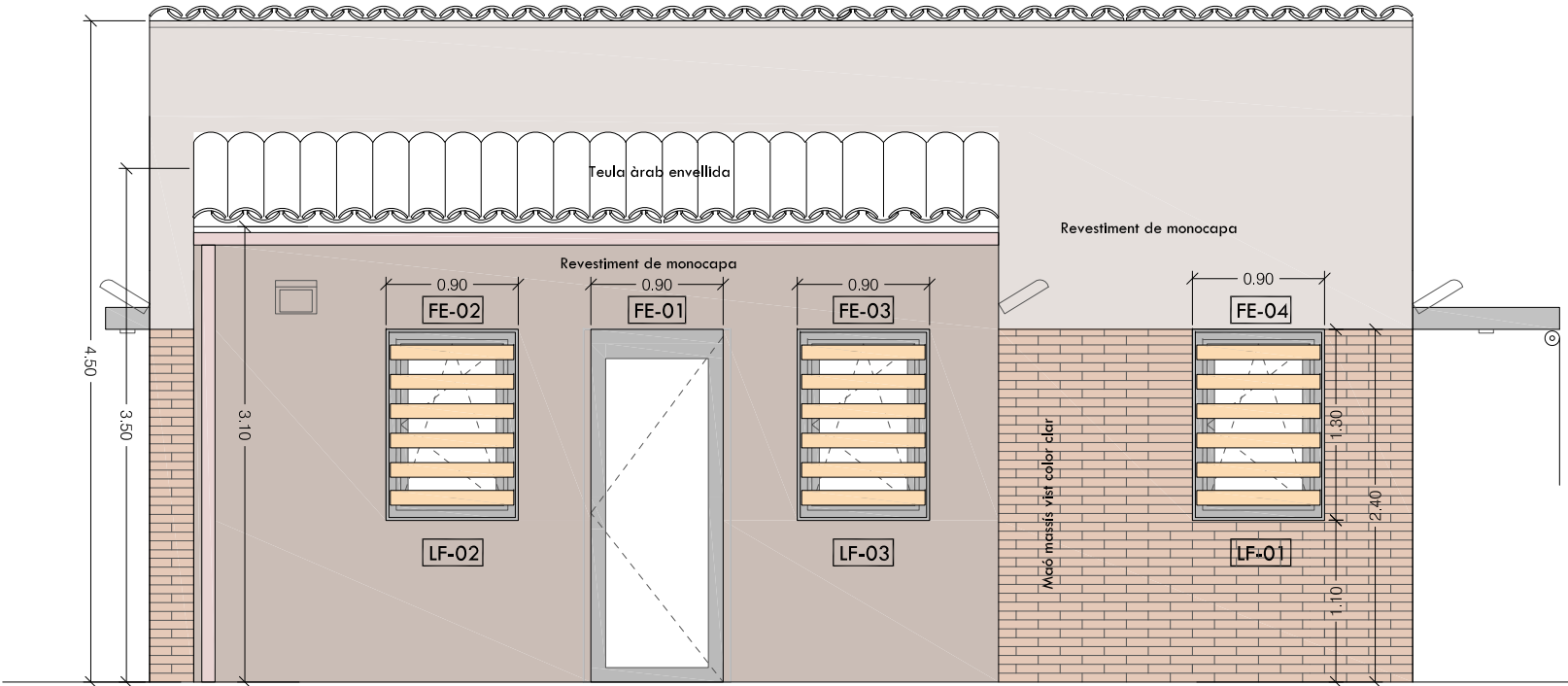
ALÇAT OEST
