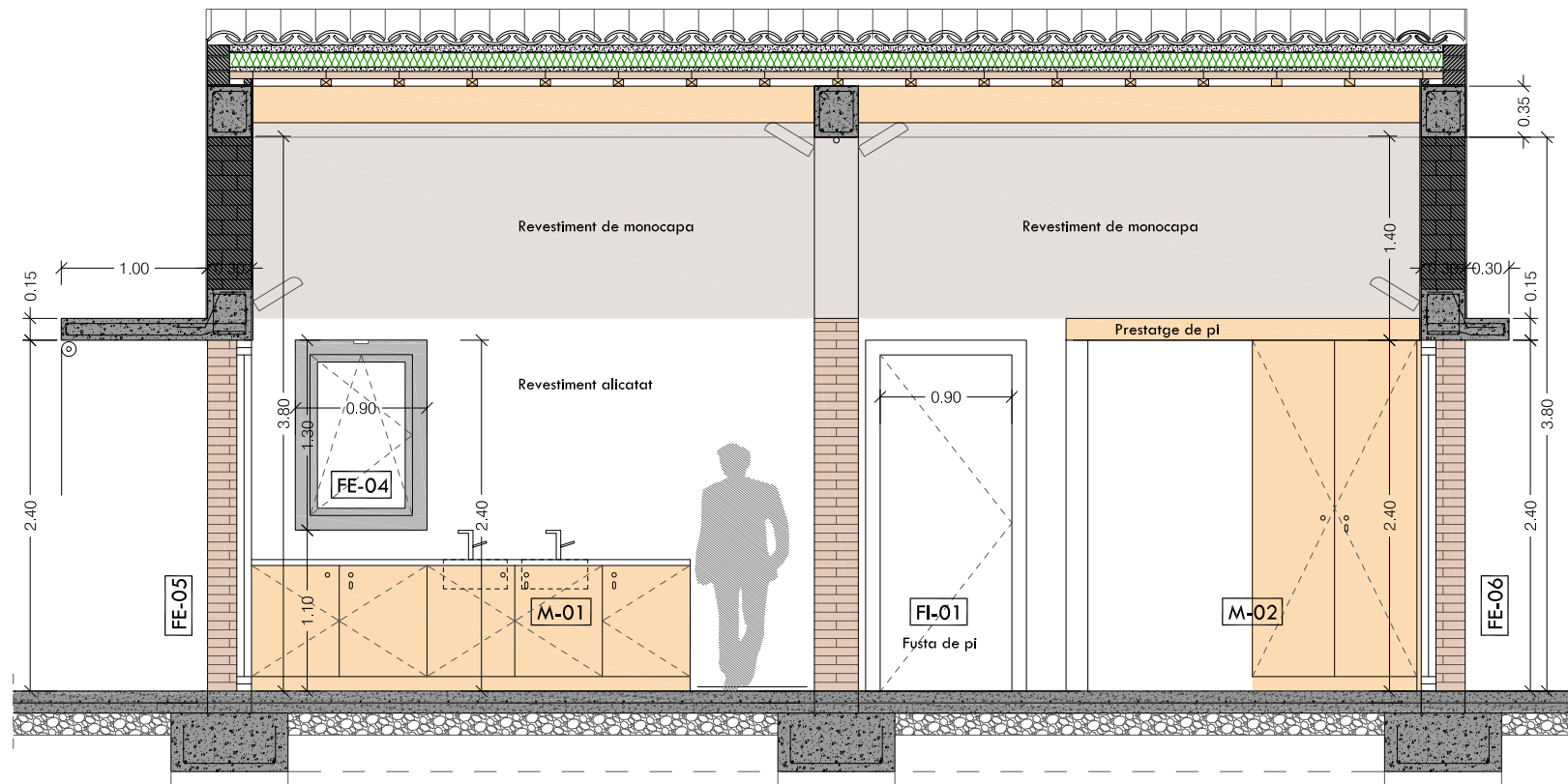
SECCIÓ LONGITUDINAL 1
