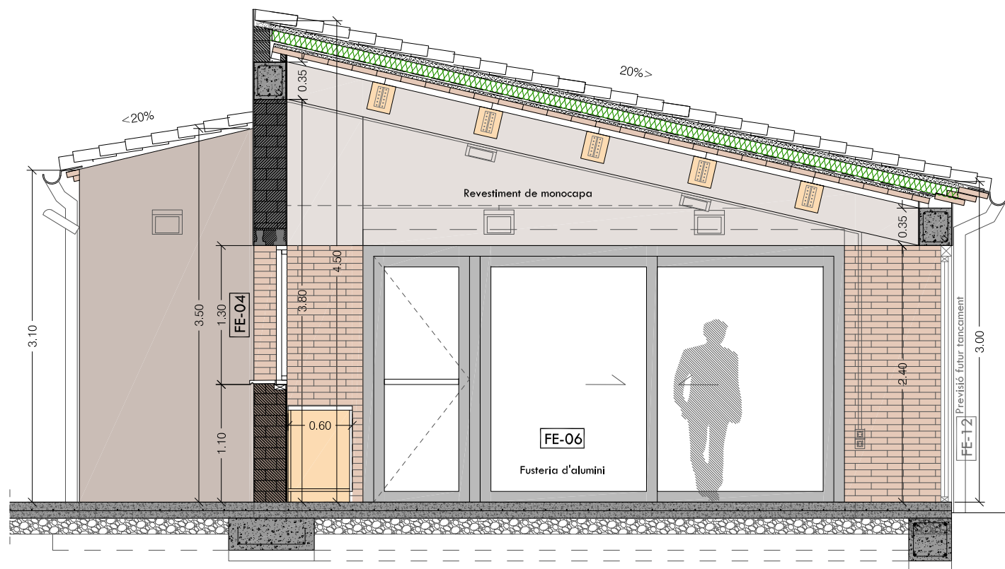
SECCIÓ TRANSVERSAL 2
