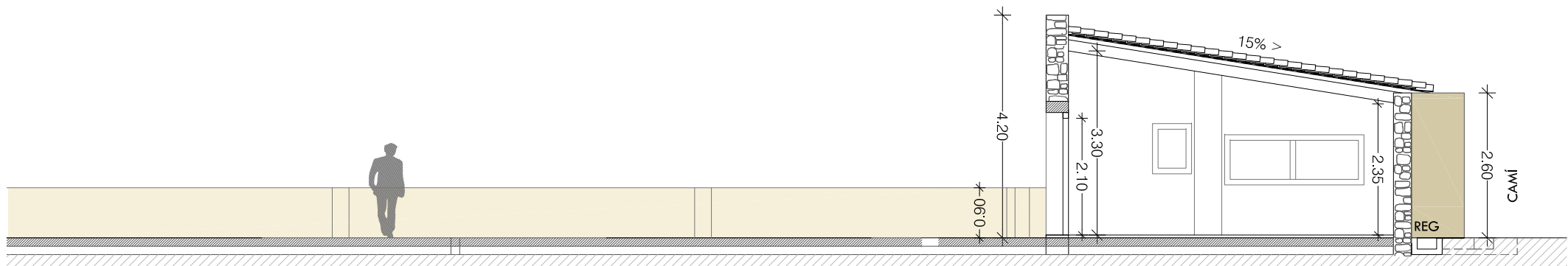
SECCIÓ 1
